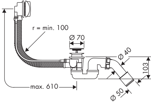
AXOR Flexaplus 58315000
