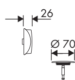
AXOR Flexaplus 58311000
