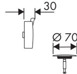
AXOR Flexaplus 58311000
