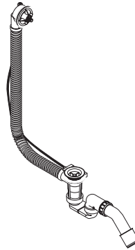
AXOR Flexaplus 58313180 / 58314180
