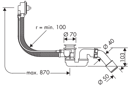
AXOR Flexaplus 58314180
