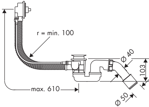
AXOR Flexaplus 58313180
